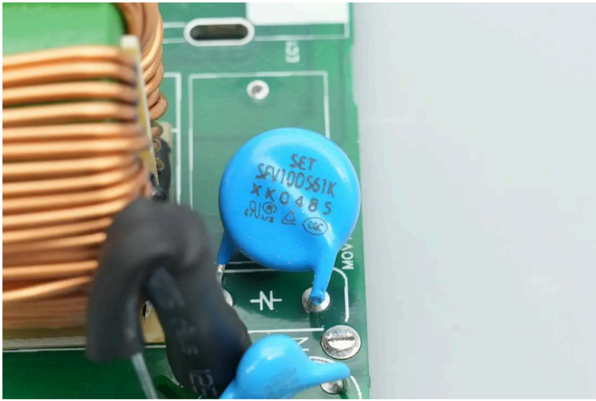
压敏电阻来自赛尔特，型号SFV10D561，用于吸收过压浪涌。
